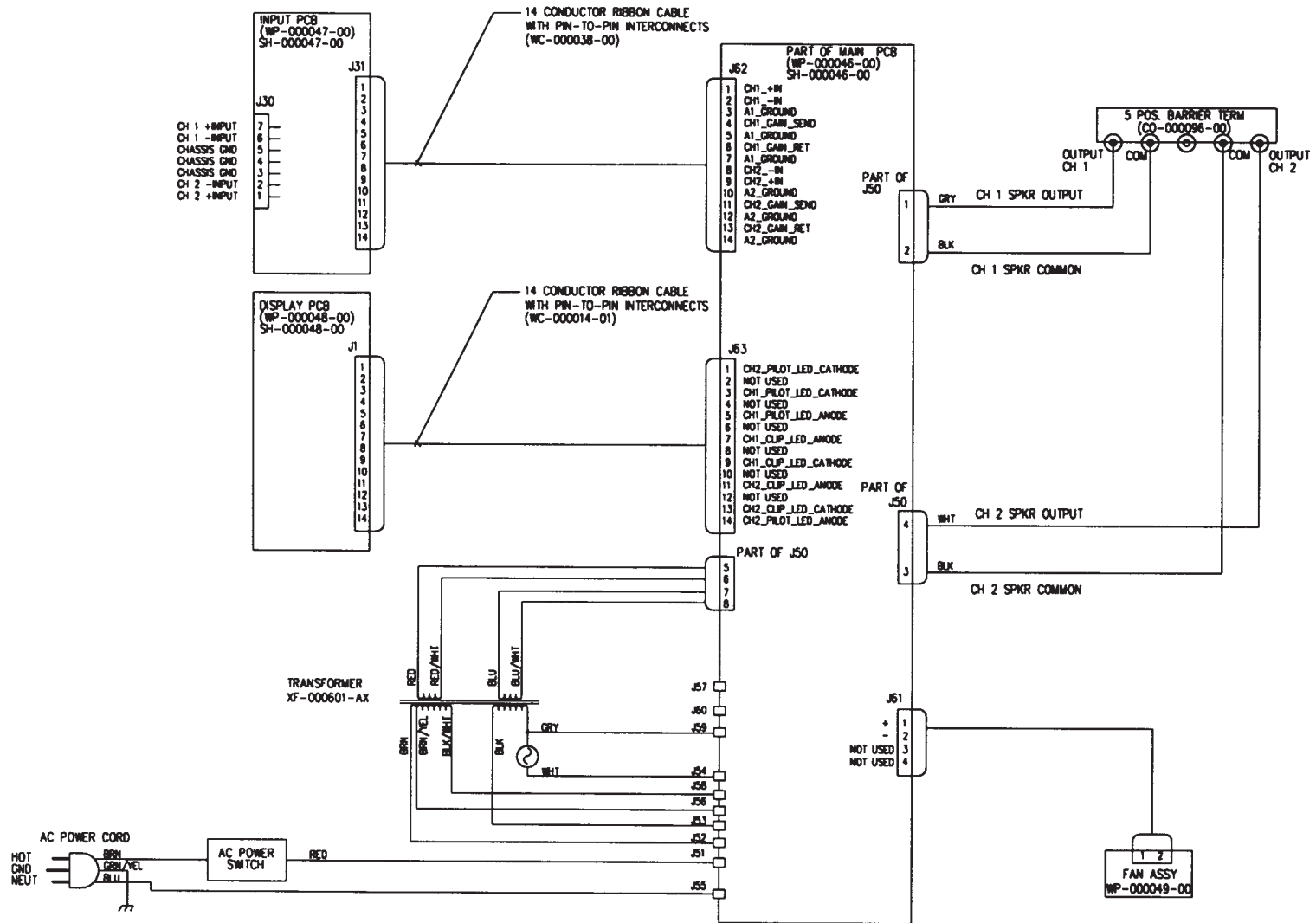
WIRING DIAGRAM, MPC200
